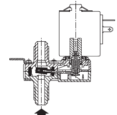
2/2 NO Function
